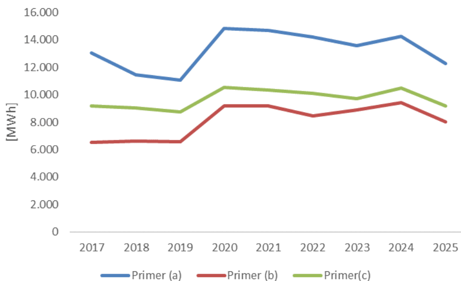
Slika 2: Potrebne povprečne dnevne količine plina za oskrbo zaščitenih odjemalcev v Republiki Sloveniji v vseh treh obravnavanih primerih po letih poročanja ( n )
